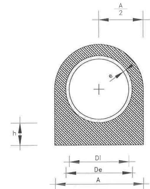
SECCION B-B
