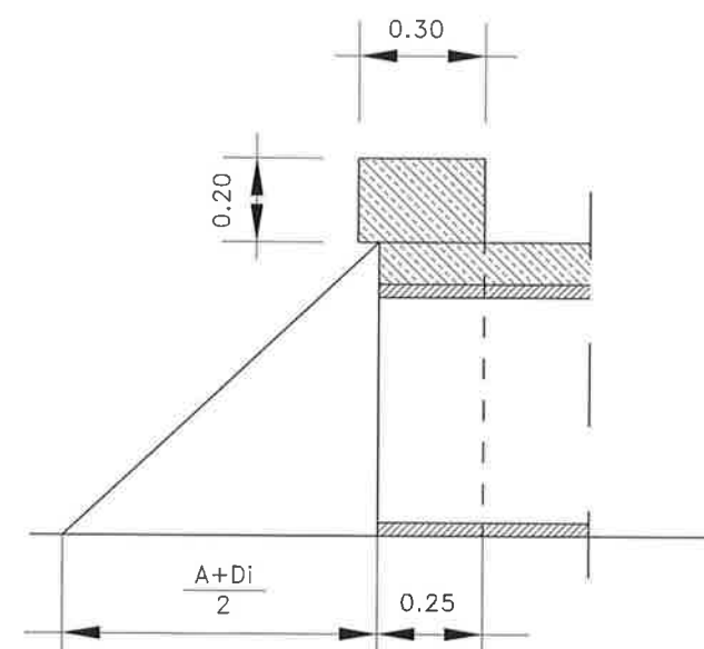
SECCION A-A
