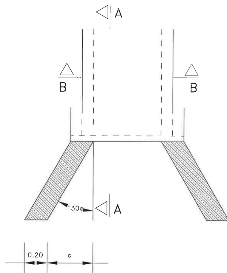
PLANTA
